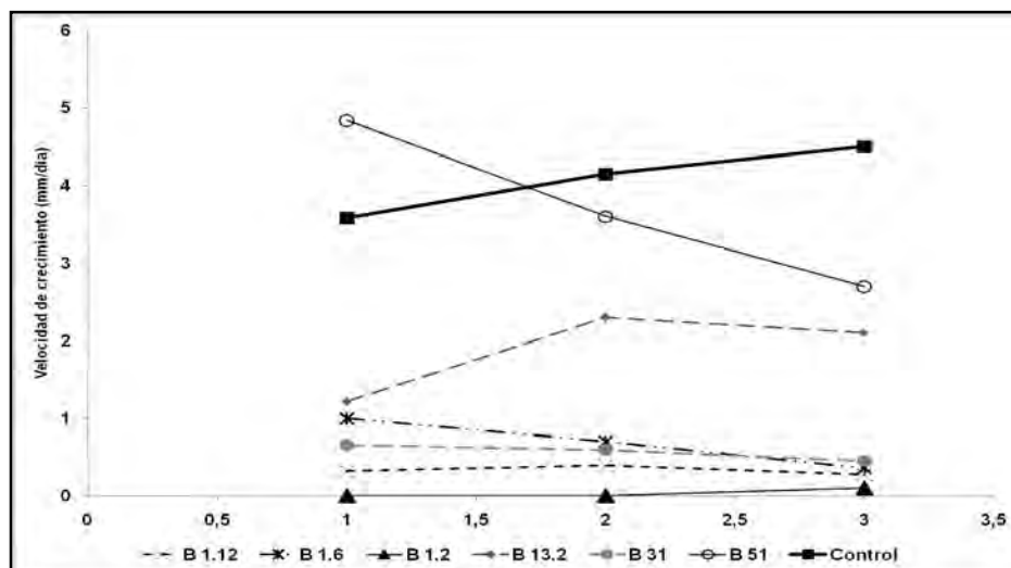
Figura 2. Velocidad de crecimiento de Cladosporium oxysporum frente a las suspensiones acuosas de las cepas.
