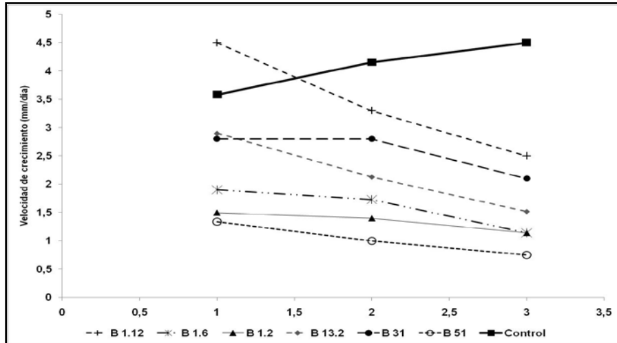
Figura 3. Velocidad de crecimiento de Cladosporium oxysporum frente a los Metabolitos Termoestables.
