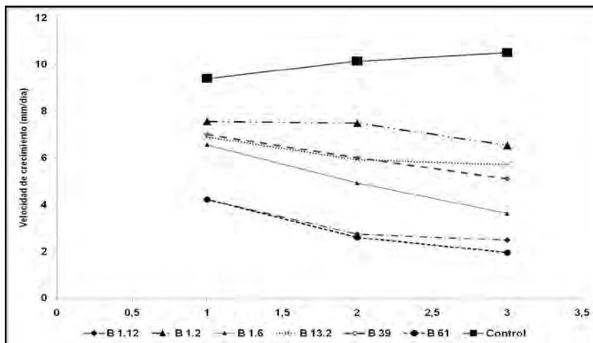
Figura 7. Velocidad de crecimiento de Fusarium oxysporum f.sp. lycopersici frente a los metabolitos termoestables.
