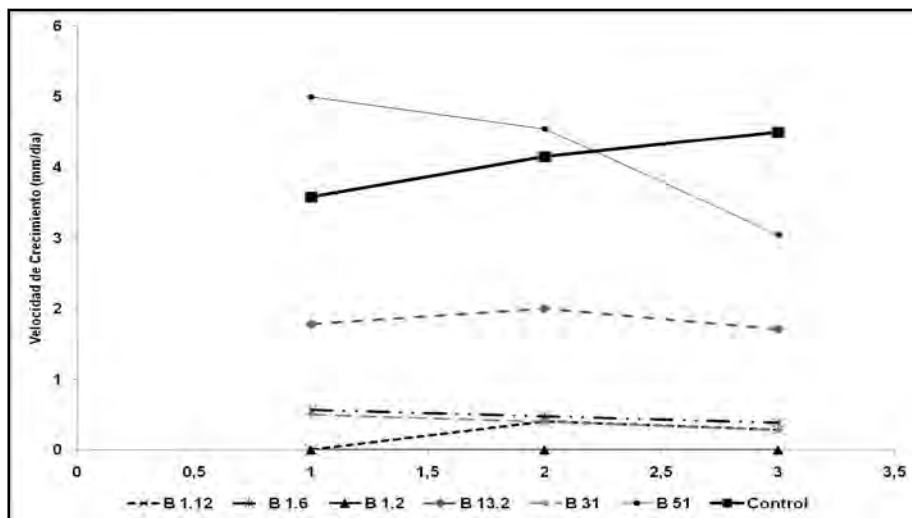
Figura 4. Velocidad de crecimiento de los Productos Viables contra Cladosporium oxysporum .
