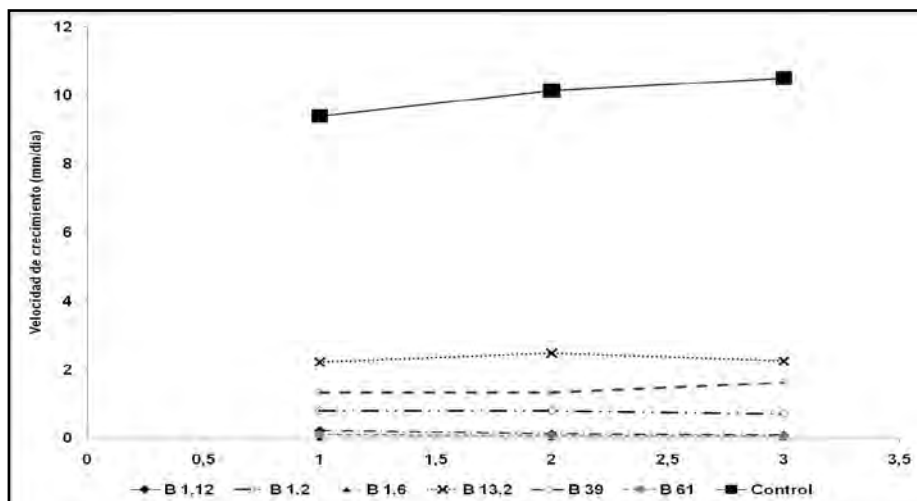
Figura 8. Velocidad de crecimiento de Fusarium oxysporum f.sp. lycopersici frente a los productos viables.
