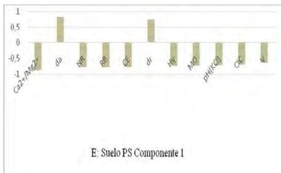
Figura 1.- Componentes principales y valores propios de los suelos estudiados. Suelo FRO (Ferrítico Rojo Oscuro Variabilidad Total: 54.83%), Suelo FRO (Ferralítico Rojo Variabilidad Total: 57.29%), Suelo PS (Pardo Sialítico Variabilidad Total: 73.52%).
