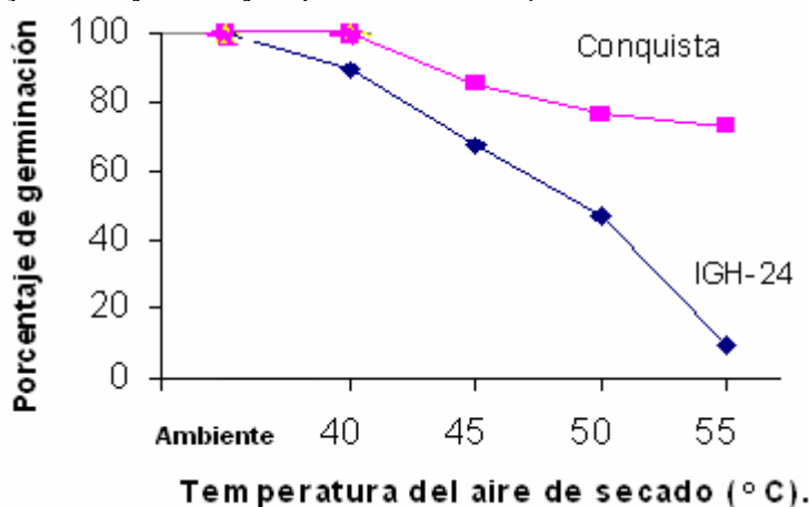
Fig. 3. Efecto de la temperatura de secado sobre la germinación de la semilla de 2 variedades de soya cultivadas en La Habana.
