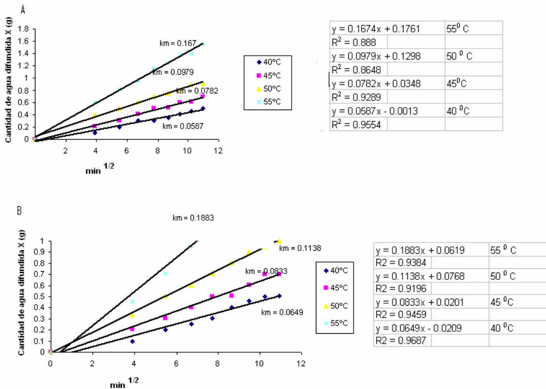
Figura 1. Relación entre la constante de difusión y la temperatura de secado de las variedades A) IGH-24 y B) Conquista. km: constante de difusión (g.m 1/2 x 10 -2 )
