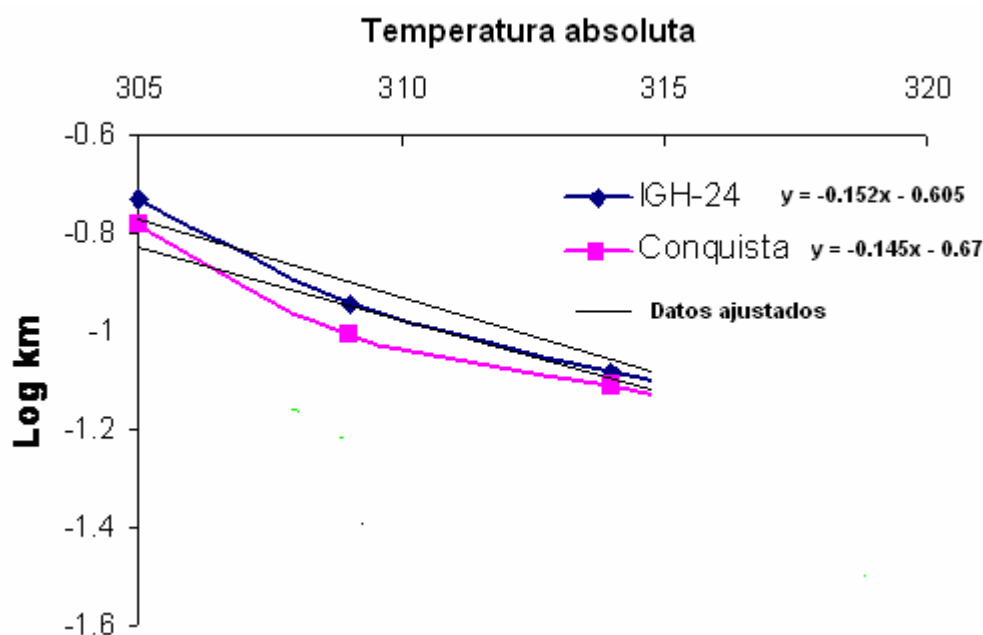
Figura 2. Influencia de la temperatura sobre la constante de difusión del agua en el grano de soya. Ecuación de Arrhenius
