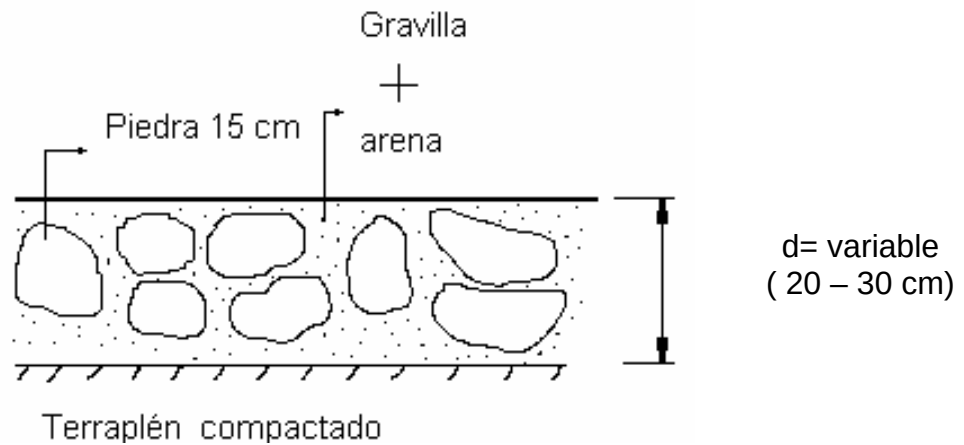
Figura 2: Capa de revestimiento propuesta para la construcción de los caminos en el área.
